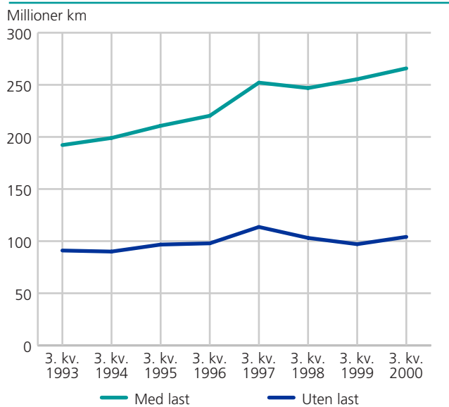
Kjøretøykilometer med og uten last. 3. kvartal. 1993-2000. Millioner km
