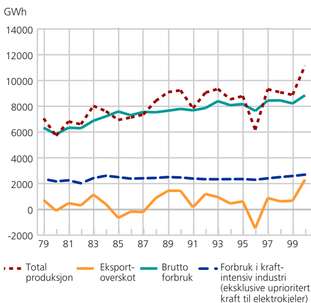
Produksjon, forbruk og eksportoverskudd av elektrisk kraft i september. 1979-2000. GWh
