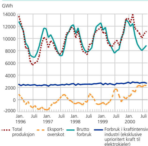
Produksjon, forbruk og eksportoverskot av elektrisk kraft per måned. GWh
