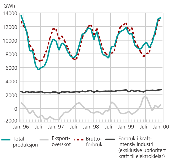
Produksjon, forbruk og eksportoverskot av elektrisk kraft per måned. GWh
