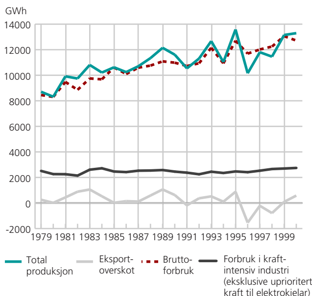
Produksjon, forbruk og eksportoverskot av elektrisk kraft i januar. 1979-2000. GWh
