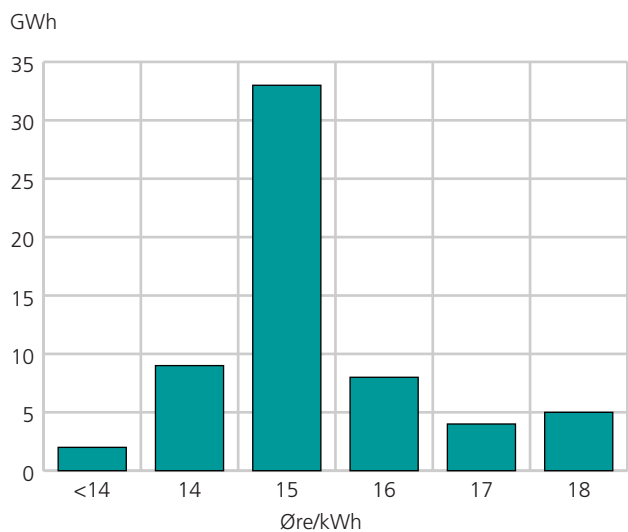
Fordeling av priser på elektrisk kraft til husholdninger, eksklusive avgifter. 4. kvartal 1999. Variabel pris, ikke tilknyttet elspot (det mest vanlige). Øre/kWh
