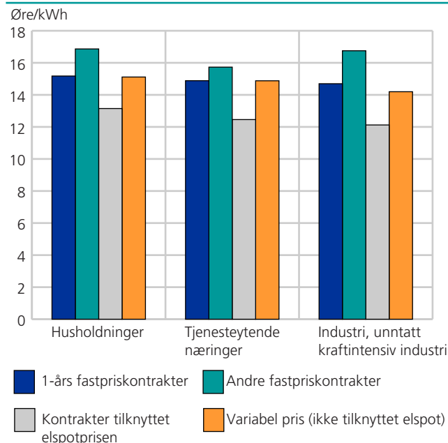
Priser på elektrisk kraft, eksklusive avgifter. Alle typer kontrakter. Gjennomsnitt for 1999. Øre/kWh
