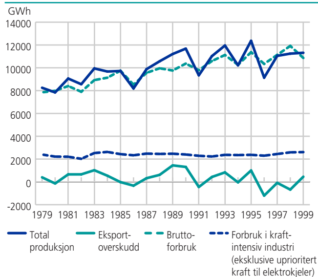
Produksjon, forbruk og eksportoverskudd av elektrisk kraft i november. 1979-1999. GWh
