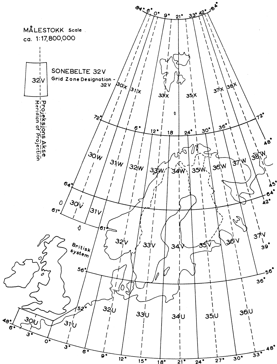
Figur 1. UTM-soner Skandinavia-Svalbard 32V: Utvidet vest til 3^{\circ} øst Greenwich Svalbard: Utvidete soner mellom 72^{\circ} N og 84^{\circ} N
