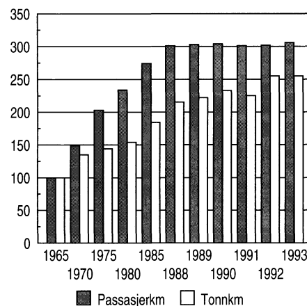
Innenlandsk transportarbeid. 1965-1993. 1965=100
