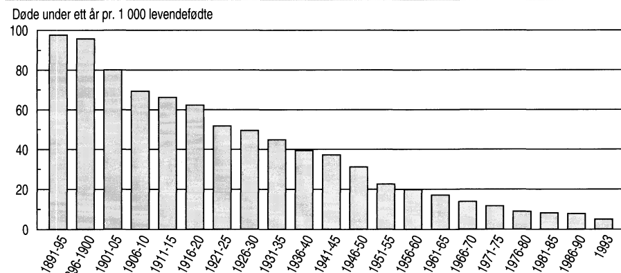
Spedbarnsdødelighet. 1891-1993
