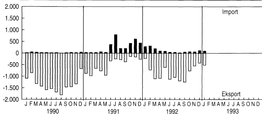
Import og eksport av elektrisk kraft. Måned. GWh
