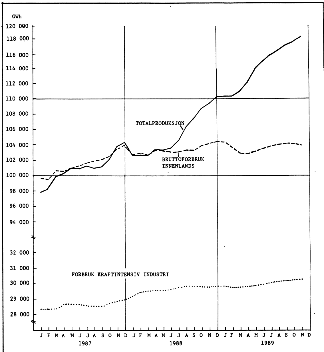
Figur 1. Produksjon, bruttoforbruk, forbruk i kraftintensiv industri. Tolvmånedersperioder
