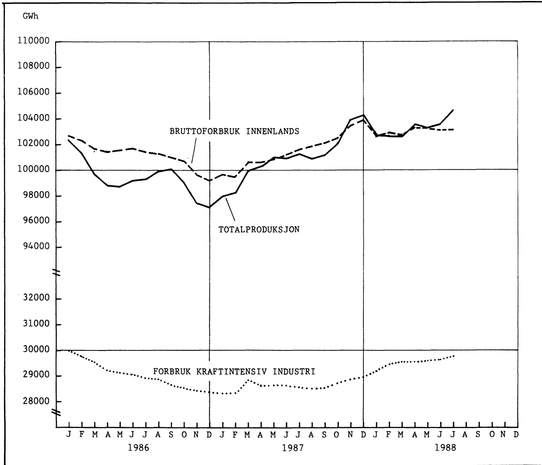
Figur 1. Produksjon, bruttoforbruk, forbruk i kraftintensiv industri. Tolvmånedersperioder
