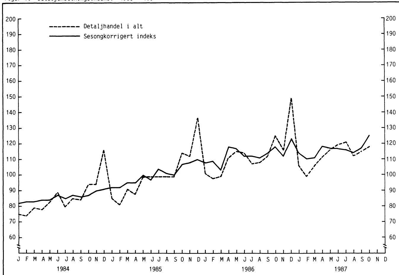
Figur 1. Detaljomsetningsindeks. 1985 = 100
