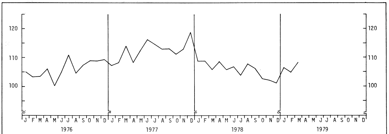
Figur 9. Detaljomsetningsvolum. Sesongkorrigert. 1975 = 100
