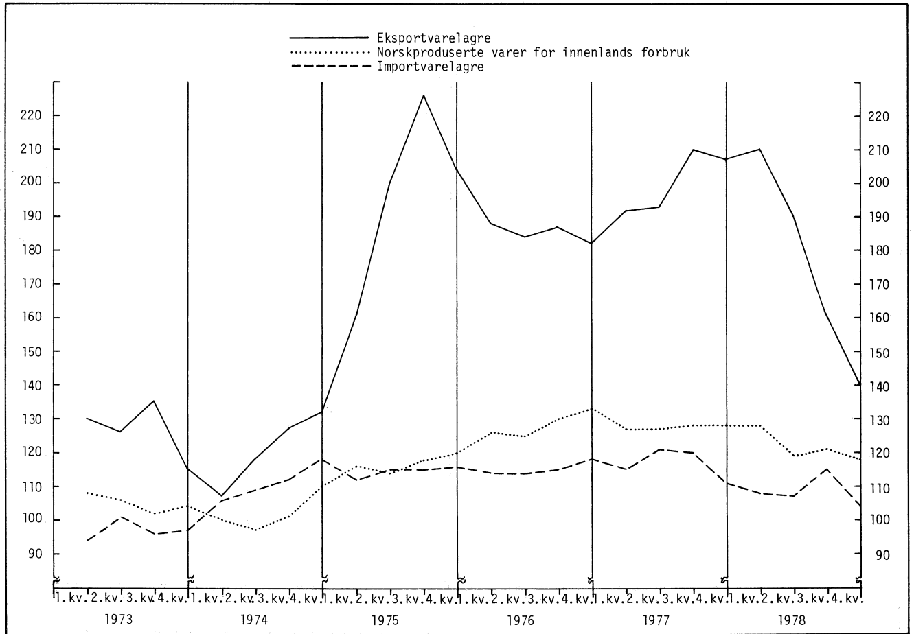
Figur 8. Lagervolum. 1970 = 100
