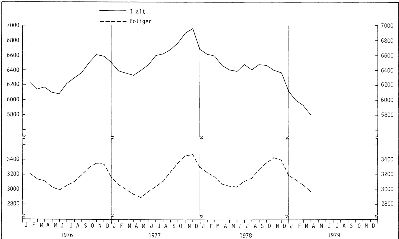
Figur 7. Bygg i arbeid. 1 000 m 2
