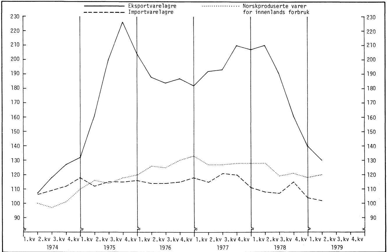
Figur 8. Lagervolum. 1970 = 100
