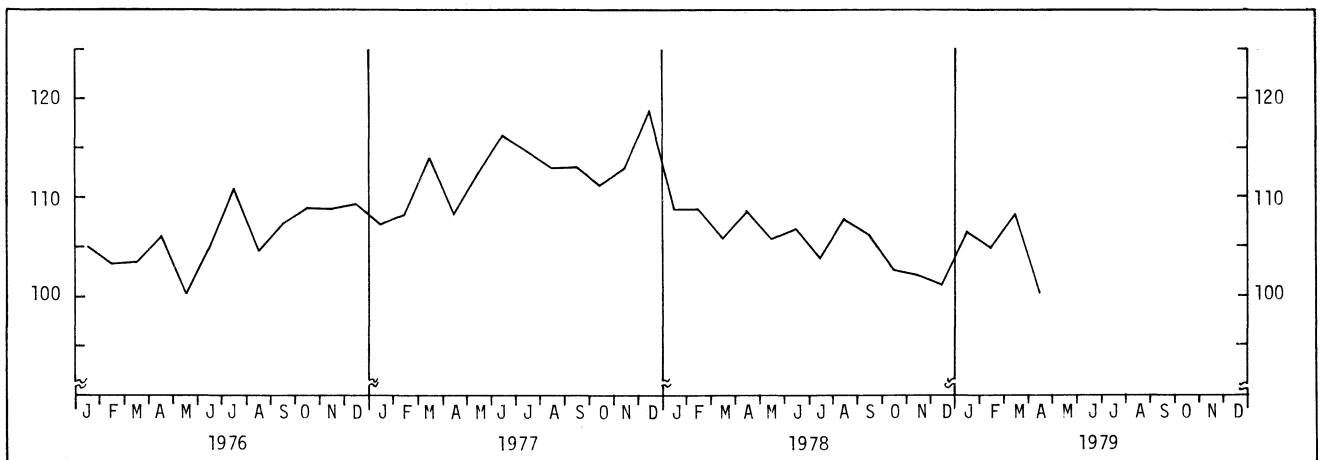
Figur 9. Detaljomsetningsvolum. Sesongkorrigert. 1975 = 100
